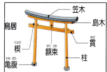
鳥居の構造と名称
